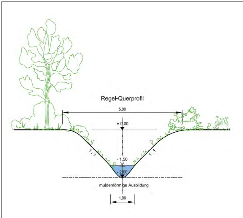
Abbildung 31: Detail zur geplanten Profilierung des „Volkerser Wassers“ (Quelle: INGENIEURBÜRO FÜR BAUWESEN DIPL.ING. (FH) STEFFEN RUPPE, Abbildung unmaßstäblich)
